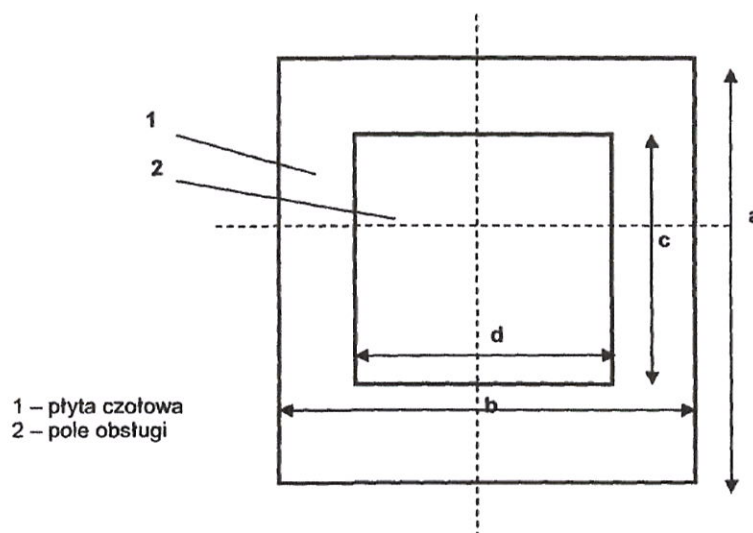
Rys. 3. Wymiary przycisku PWP
