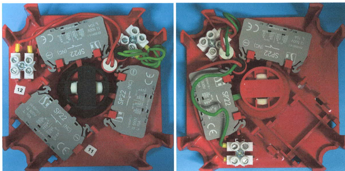
Rys. 2. Wnętrze ręcznego przycisku przeciwpożarowego wyłącznika prądu typu PWP1 w odmianach PWP1-W01-A-03-2LED7 i PWP1-W01-B-11-2LED11
